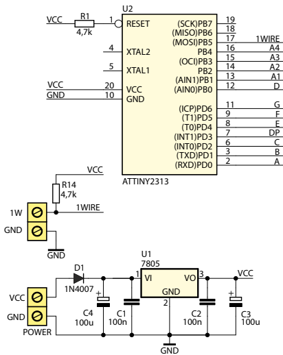
Rys. 1. Schemat ideowy
