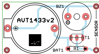
Rys. 2. Rozmieszczenie elementów na płytce drukowanej
