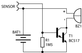
Rys. 1. Schemat ideowy
